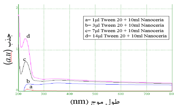
شکل ۴: طیف جذبی نانوذرات سربیم اکساید در حضور غلظت‌های مختلف از سوفکتانت غیریونی توپین ۲۰ (Tween 20)
