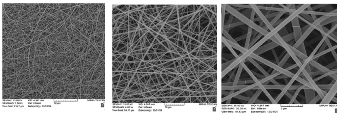
شکل ۳: تصاویر SEM تهیه شده از بسترهای PDLLA الکترونیسی شده در شرایط بهینه
