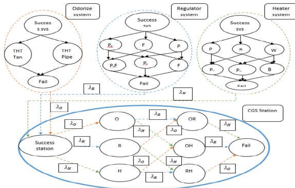
شکل ۱۲: رویکرد سیستماتیک بر اساس مدل مارکوف برای ایستگاه تقلیل فشار ۱۱
