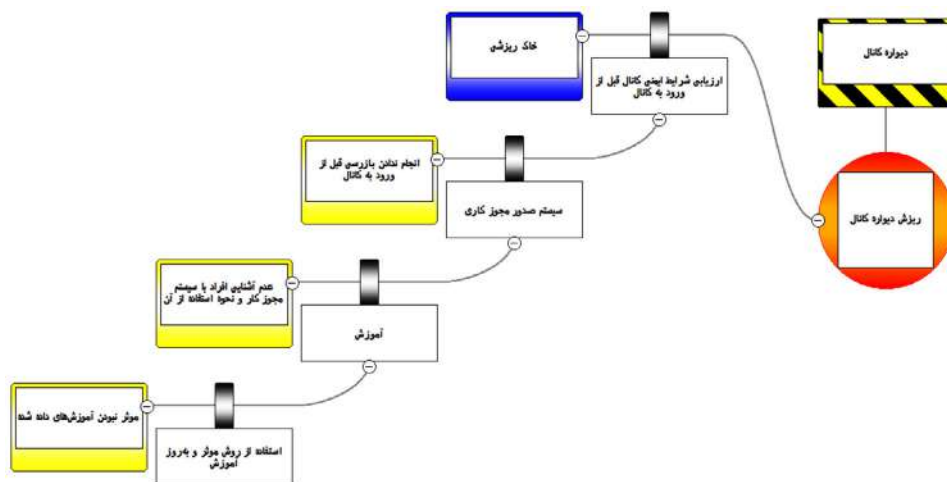
شکل ۱۰: نمودار Bowtie برای فاکتور تشدید کننده سیستم صدور مجوز کاری در حوادث ریش دیواره کانال در عملیات گودبرداری و لوله‌گذاری خطوط لوله گاز
