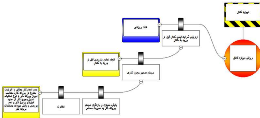
شکل ۱۳: نمودار Bowtie برای فاکتور تشدید کننده سیستم صدور مجوز کاری در حوادث ریزش دیواره کانال در عملیات گودبرداری و لوله‌گذاری خطوط لوله گاز
