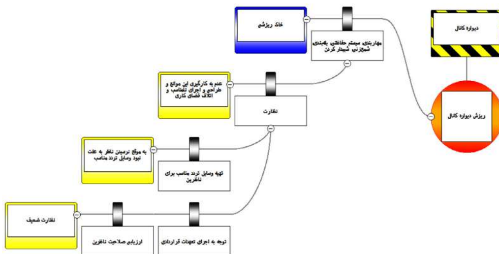
شکل ۹: نمودار Bowtie برای فاکتورهای تشدید کننده نظارت در حوادث ریزش دیواره کانال در عملیات گودبرداری و لوله‌گذاری خطوط لوله گاز
