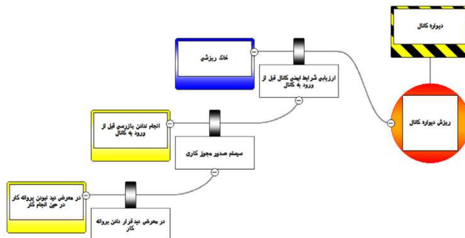
شکل ۱۲: نمودار Bowtie برای فاکتور تشدید کننده سیستم صدور مجوز کاری در حوادث ریش دیواره کانال در عملیات گودبرداری و لوله‌گذاری خطوط لوله گاز
