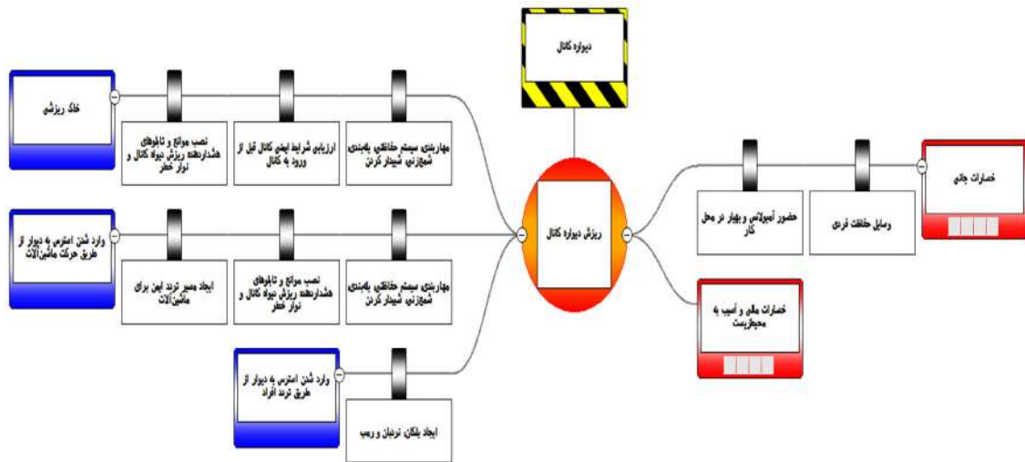
شکل ۳: نمودار Bowtie برای حوادث ریزش دیواره کانال در عملیات گودبرداری و لوله‌گذاری خطوط لوله گاز
