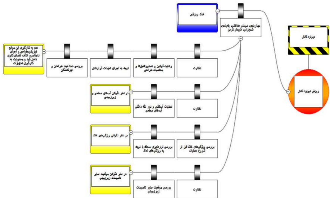
شکل ۴: نمودار Bowtie برای فاکتورهای تشدید کننده سیستم‌های حفاظتی در حوادث ریزش دیواره کانال در عملیات گودبرداری و لوله‌گذاری خطوط لوله گاز
