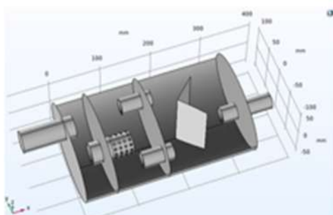
مدل CAD مافلر B یا طول لوله رابط ۶mm و سوراخدار
