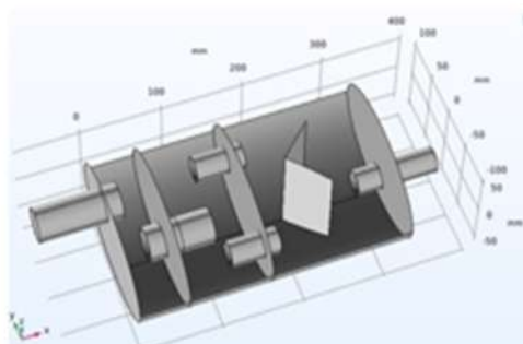
مدل CAD مافلر E یا طول لوله رابط ۶mm و بدون سوراخ
