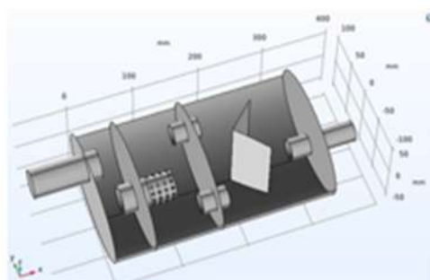
مدل CAD مافلر A یا طول لوله رابط ۴mm و سوراخدار
