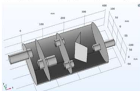
مدل CAD مافلر D یا طول لوله رابط ۴mm و بدون سوراخ
