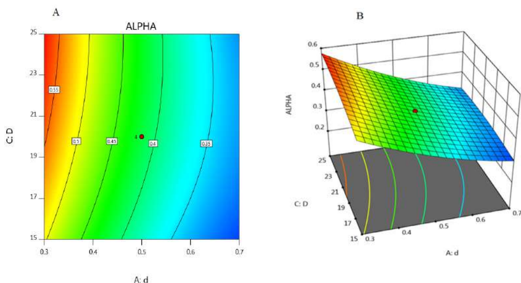
شکل ۴: نمای دو بعدی (A) و سه بعدی (B) تاثیر متغیرهای d و D بر روی ضریب جذب
