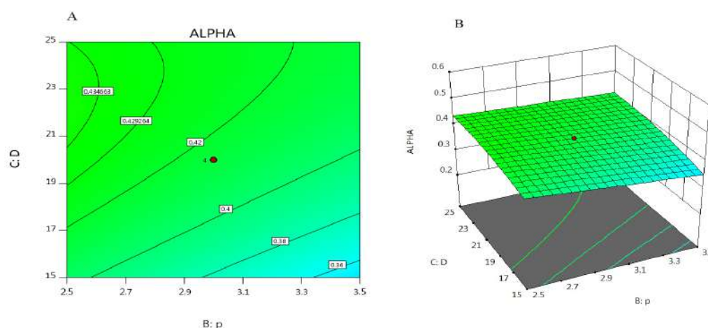
شکل ۵: دو بعدی (A) و سه بعدی (B) تاثیر متغیرهای P و D بر روی ضریب جذب
